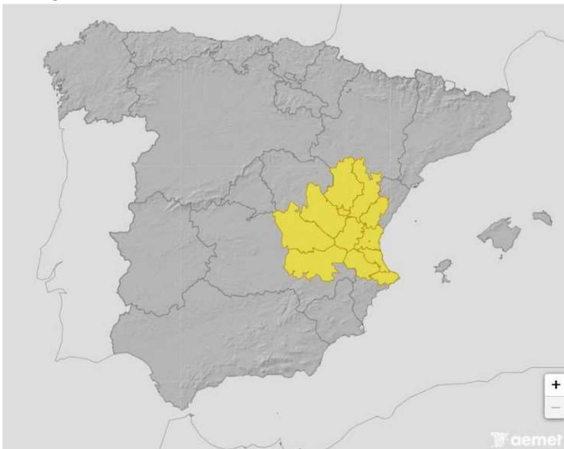
Mapa de avisos por lluvias y tormentas para el miércoles 8 de octubre*
