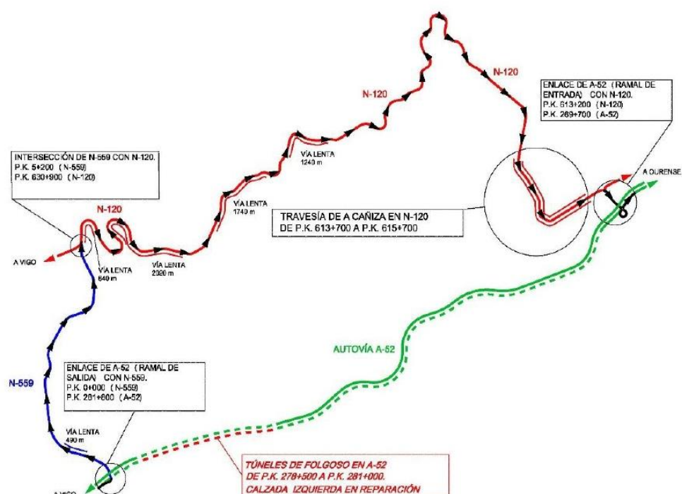
ITINERARIO ALTERNATIVO 1: CORTE DE CALZADA SENTIDO OURENSE Descargar imagen
