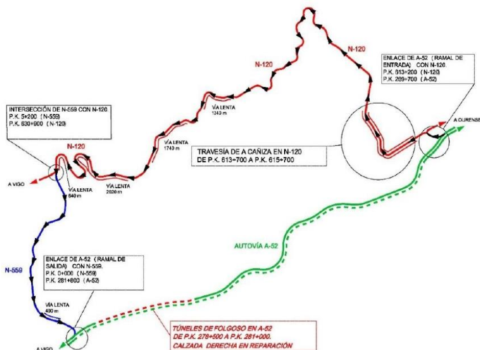
ITINERARIO ALTERNATIVO 2: CORTE DE CALZADA SENTIDO VIGO
